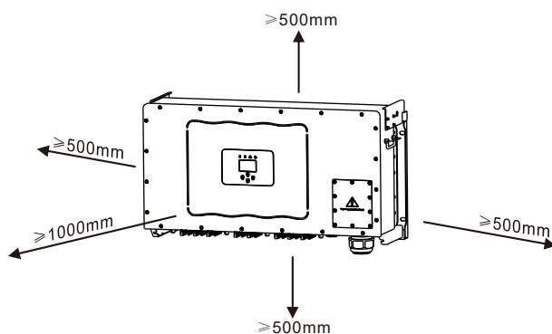
Figura 4.3 Espaço de instalação
