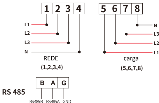
Figura 7.1 Medidor Eastron
