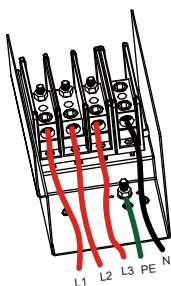
Figura 5.9 Condutor CA conectado ao terminal
