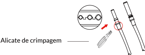
Figura 5.4 Prenda o pino de contato no fio
