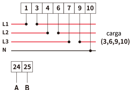
Figura 7.28 Medidor CHINT
